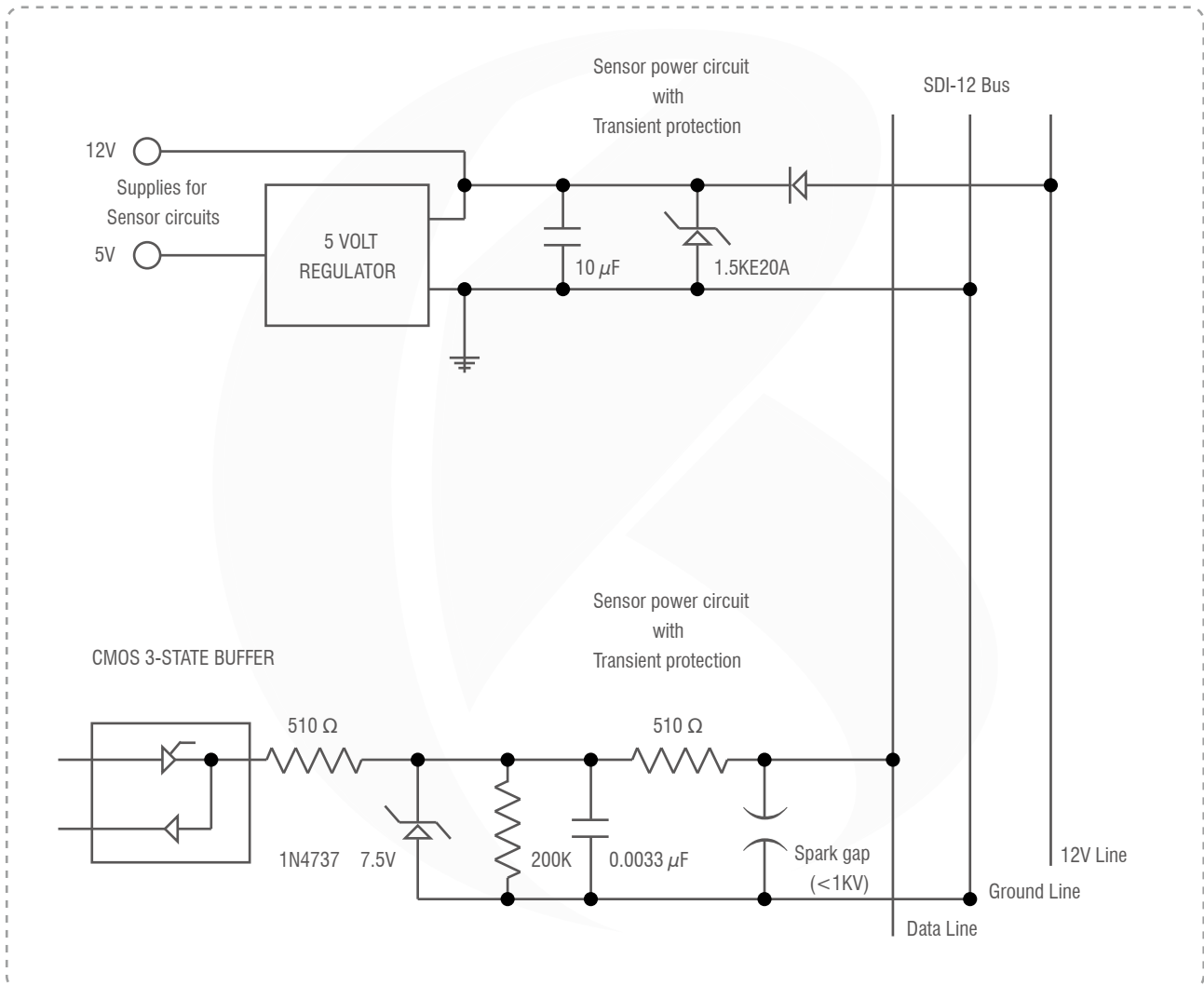
图11. SDI-12推荐电路
